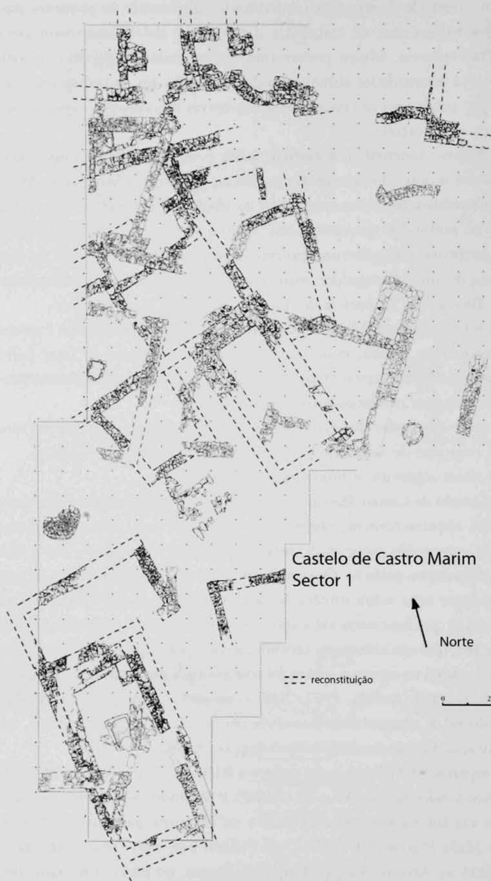
Fig. 43 – Castelo de Castro Marim – plantas das Fases IV e V sobrepostas, evidenciando a profunda alteração estrutural observada nos finais do século VI a.C.. O espaço reorganiza-se e altera-se a orientação do urbanismo.
