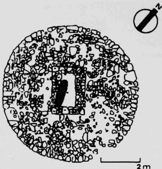
Fig. 68 – Planta do monumento funerário do Pego da Sobreira, segundo Correia, 1993.
