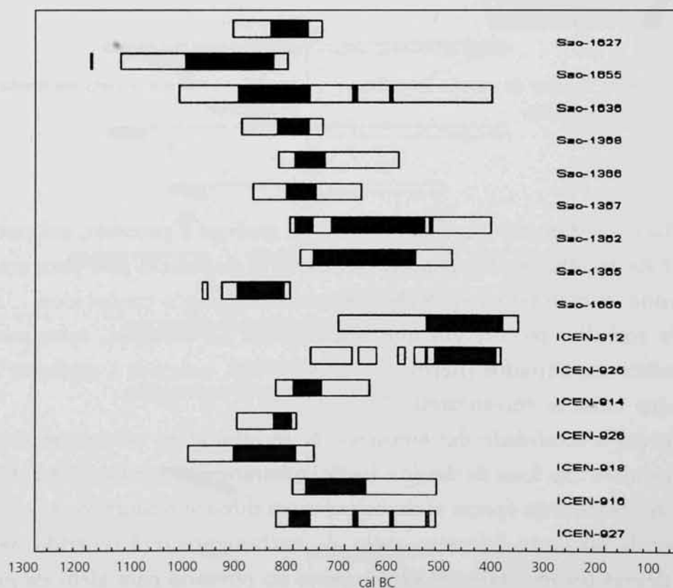
Fig. 13 – As datações de radiocarbono da Quinta do Almaraz, segundo Barros e Soares, 2004.
