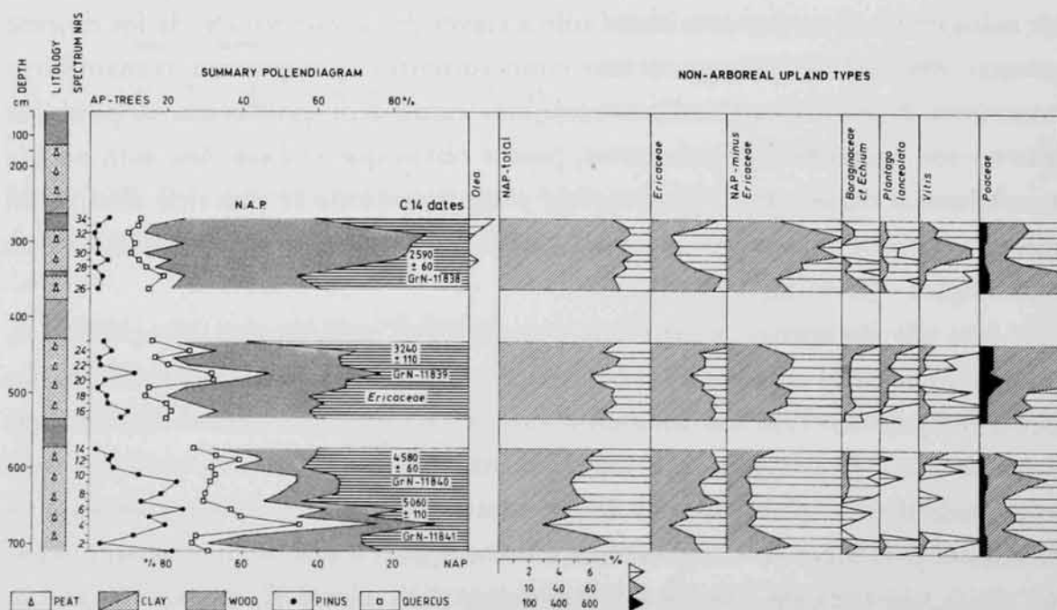
Fig. 40 – Perfis polínicos de Alpiarça, segundo Leeuwaarden e Janssen, 1985.
