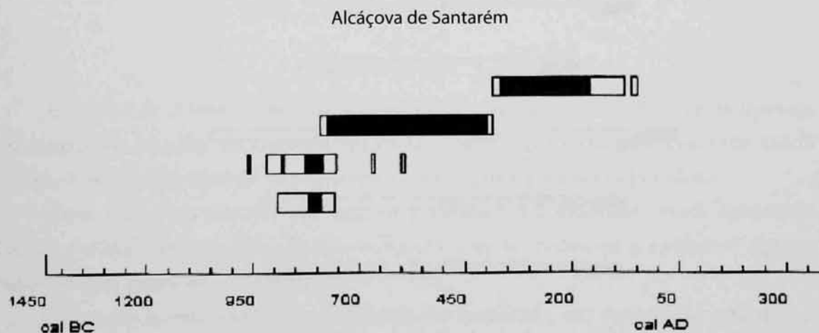
Fig. 8 – A sequência radiocarbónica de Santarém a 2 sigmas.
