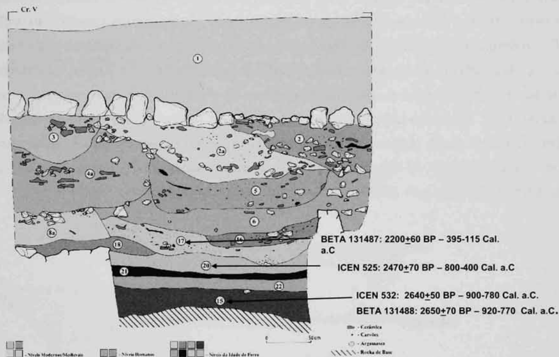
Fig. 7 – Sequência estratigráfica de Santarém, com a indicação dos níveis onde se recolheram os restos orgânicos datados pelo radiocarbono, e respectivos resultados.
