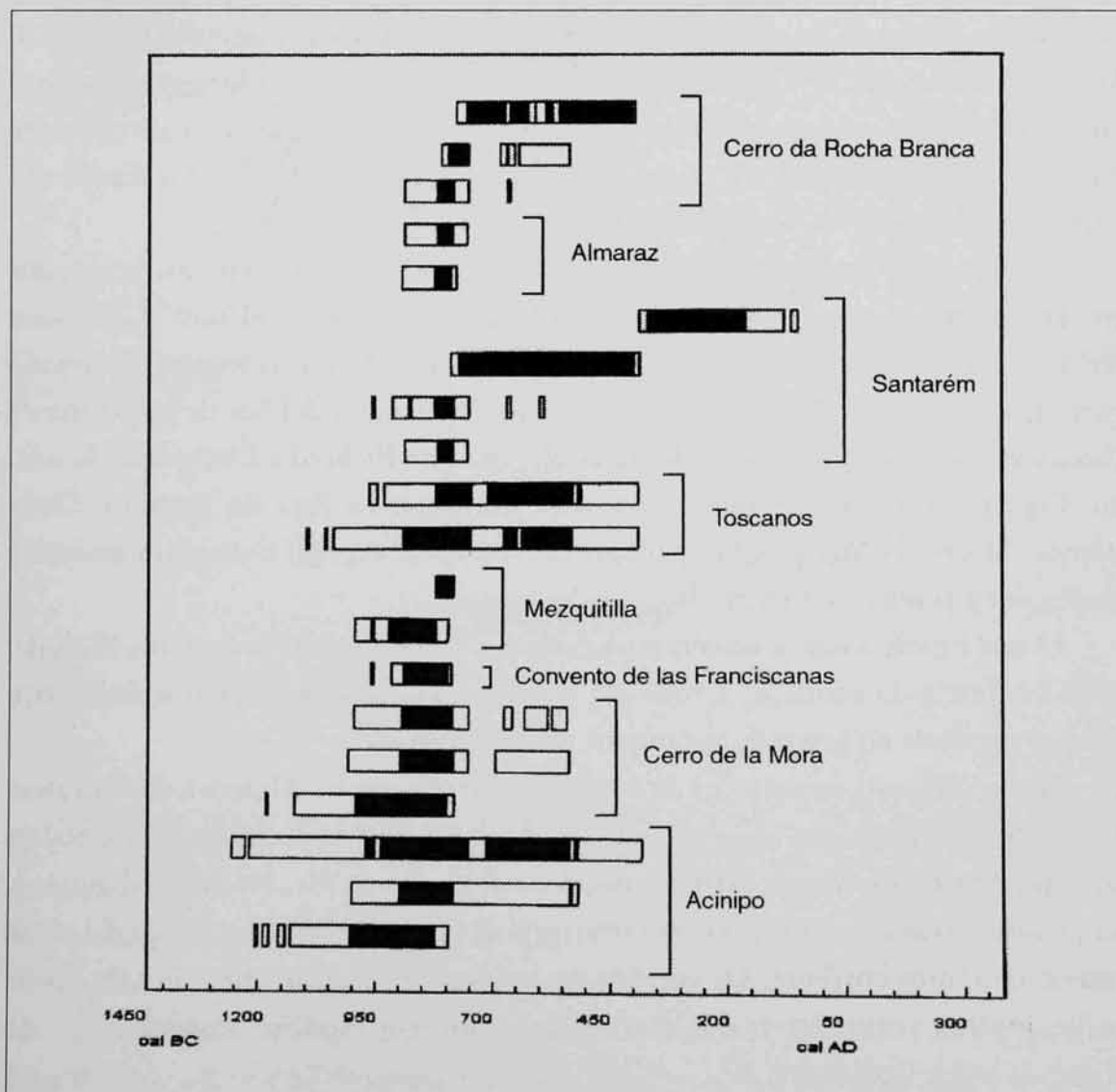
Fig. 6 - Tábua das datações de radiocarbono de sítios portugueses e espanhóis.
