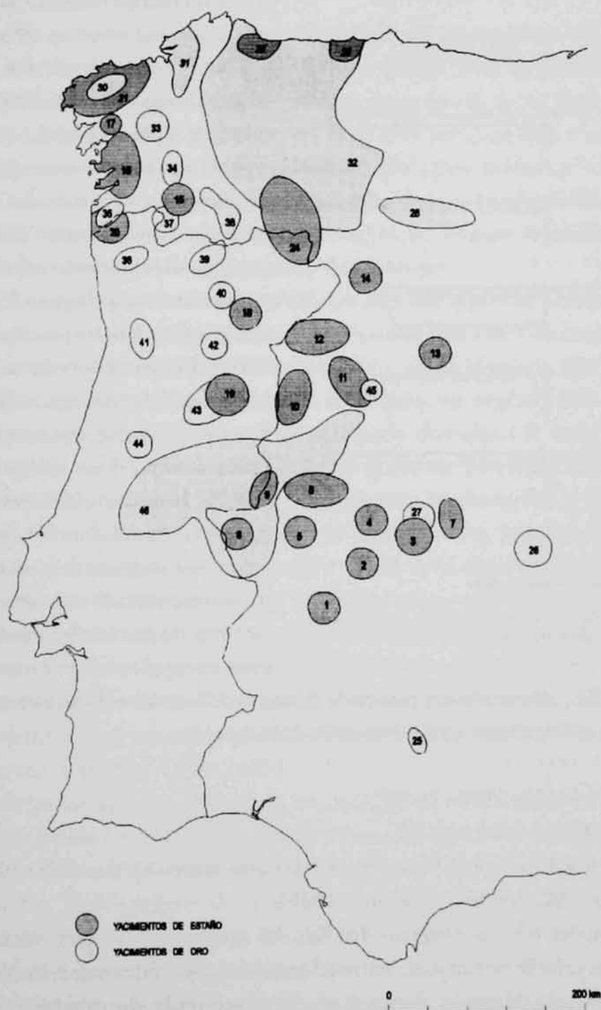
Fig. 38 – Recursos estaníferos e auríferos do Ocidente peninsular, segundo Pellicer, 2000.
