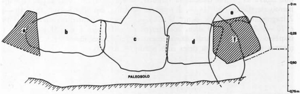
Fig.13 — Alçado da parede Norte da câmara funerária (esc. 1 : 20).
