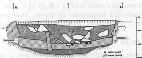
Fig. 7 — Perfil estratigráfico E.-W. (esc. 1 : 40).
