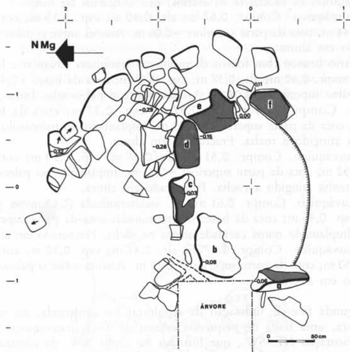
Fig. 5 — Planta do monumento (esc. 1 : 40).
