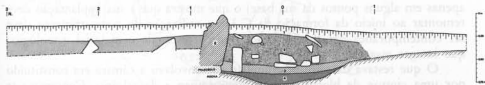
Fig. 6 — Perfil estratigráfico N.-S. (esc. 1 : 40).
